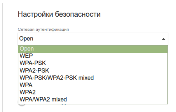
Рисунок 88. Типы аутентификации, поддерживаемые маршрутизатором.
