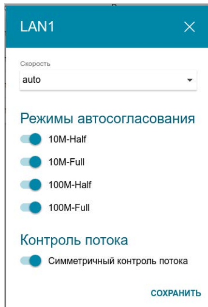
Рисунок 118. Окно изменения настроек порта маршрутизатора.
