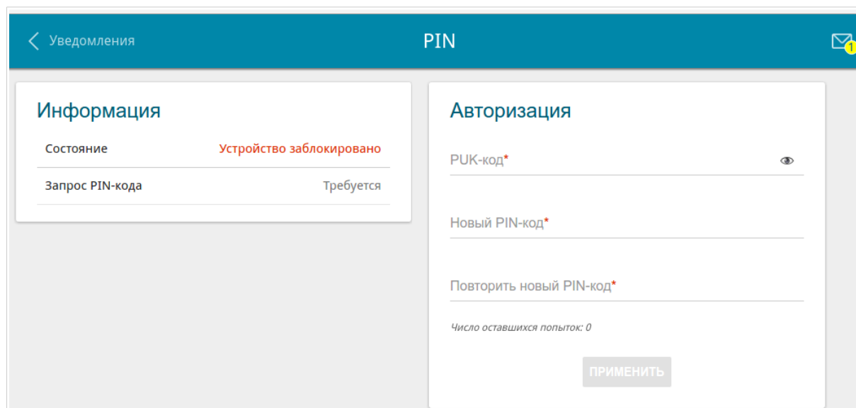
Рисунок 104. Страница LTE-модем / PIN . Запрос PUK-кода.
