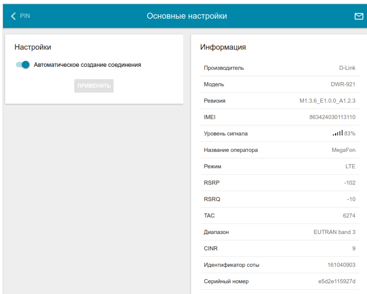
Рисунок 102. Страница LTE-модем / Основные настройки .
