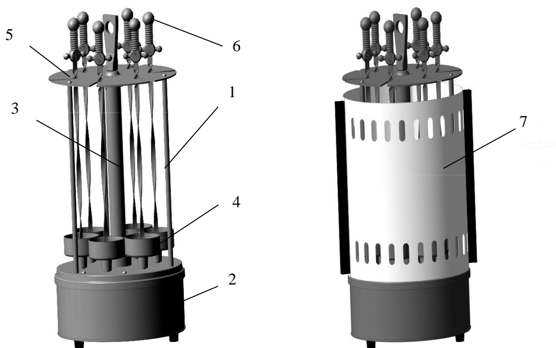
Рисунок 1 – Электрошашлычница.
